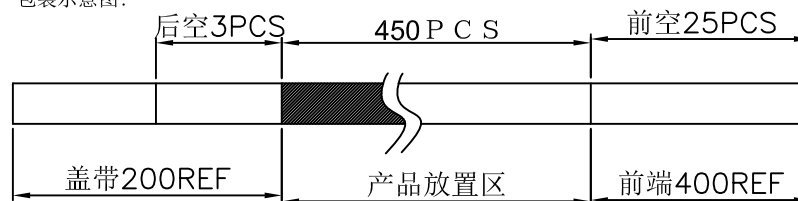
包装示意图:
