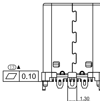
截面 A-A
